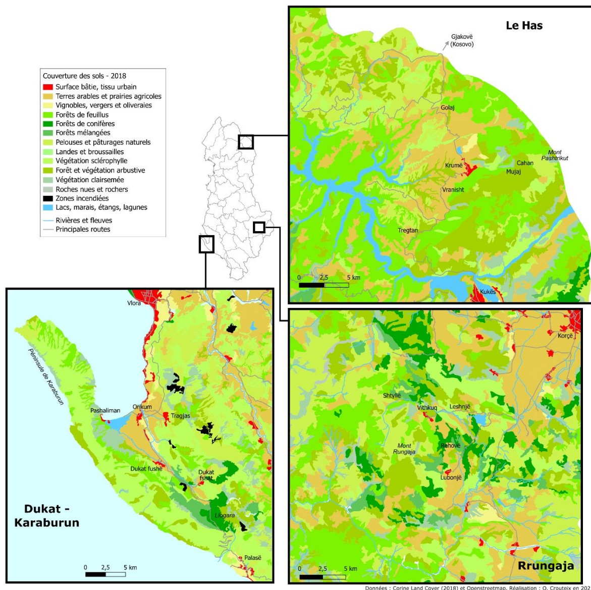
Figure 3 : les couvertures du sol en 2018 pour les trois territoires de l'étude (O. Crouteix, 2021)
